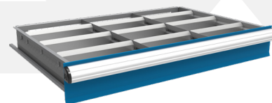
Le code du produit est : DR52436-12-0209_ (Tiroir 5"H x 24"P x 36"L - 12 compartiments)
