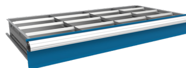
Le code du produit est : DR62448_-16-0312_ (Tiroir 6"H x 24"P x 48"L - 16 compartiments)
